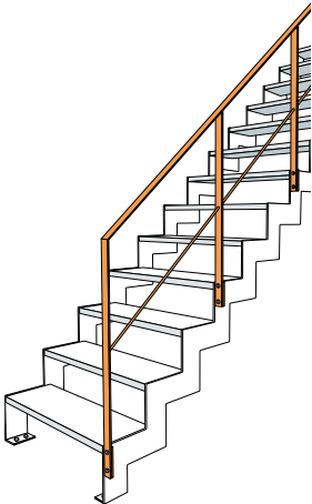
フラットバー+丸鋼
